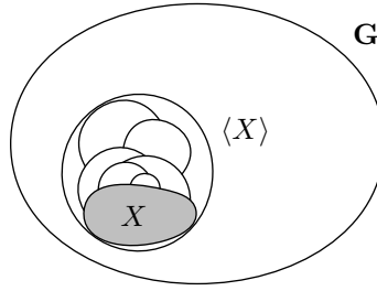
OBRÁZEK 6. Ilustrace generování podgrupy \langle X \rangle_{\mathbf{G}} .
