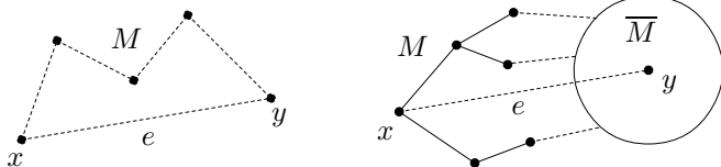
Situace v důkazu Bezbarvého lemmatu
