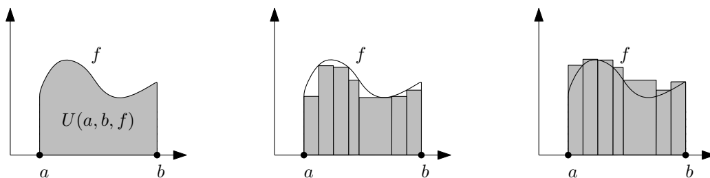
Obrázek 11.2: Oblast U(a, b, f) pod grafem funkce f (vlevo), a Riemannova metoda odhadu jejího plošného obsahu zdola (uprostřed) a shora (vpravo).
